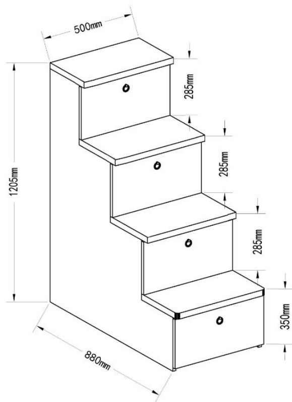
图 12：走梯尺寸图
