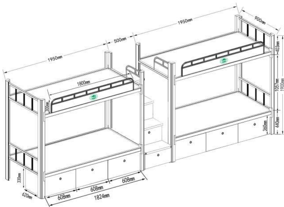
图 3：两连体四人位上下床尺寸图
