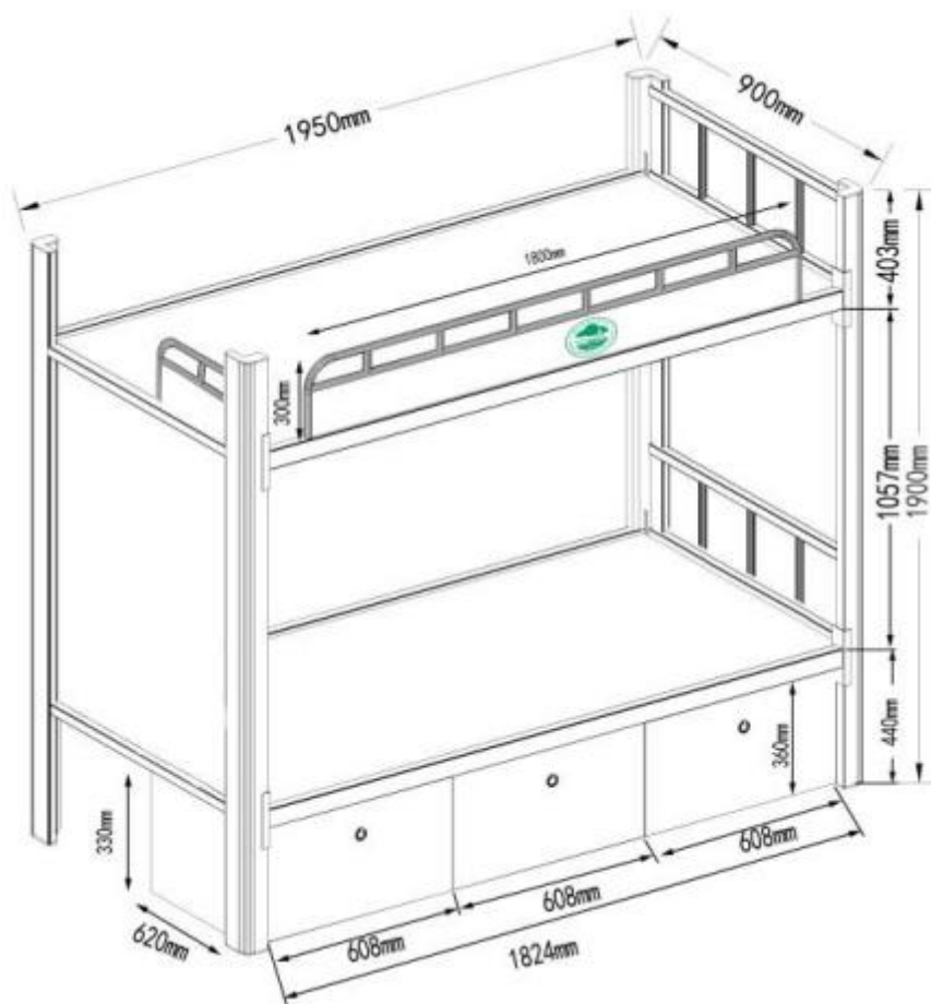
图 11：两人位上下床尺寸图
