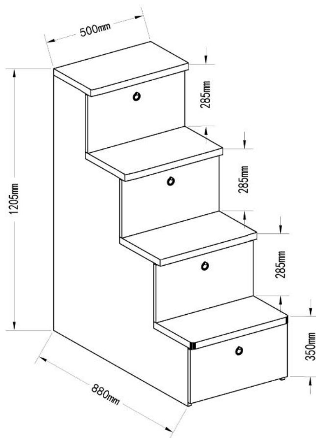
图 4：走梯尺寸图
