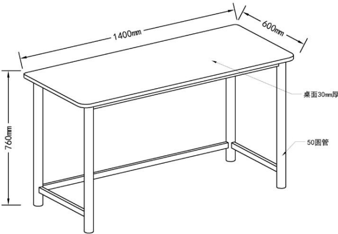
图 16：双人学习桌尺寸图
