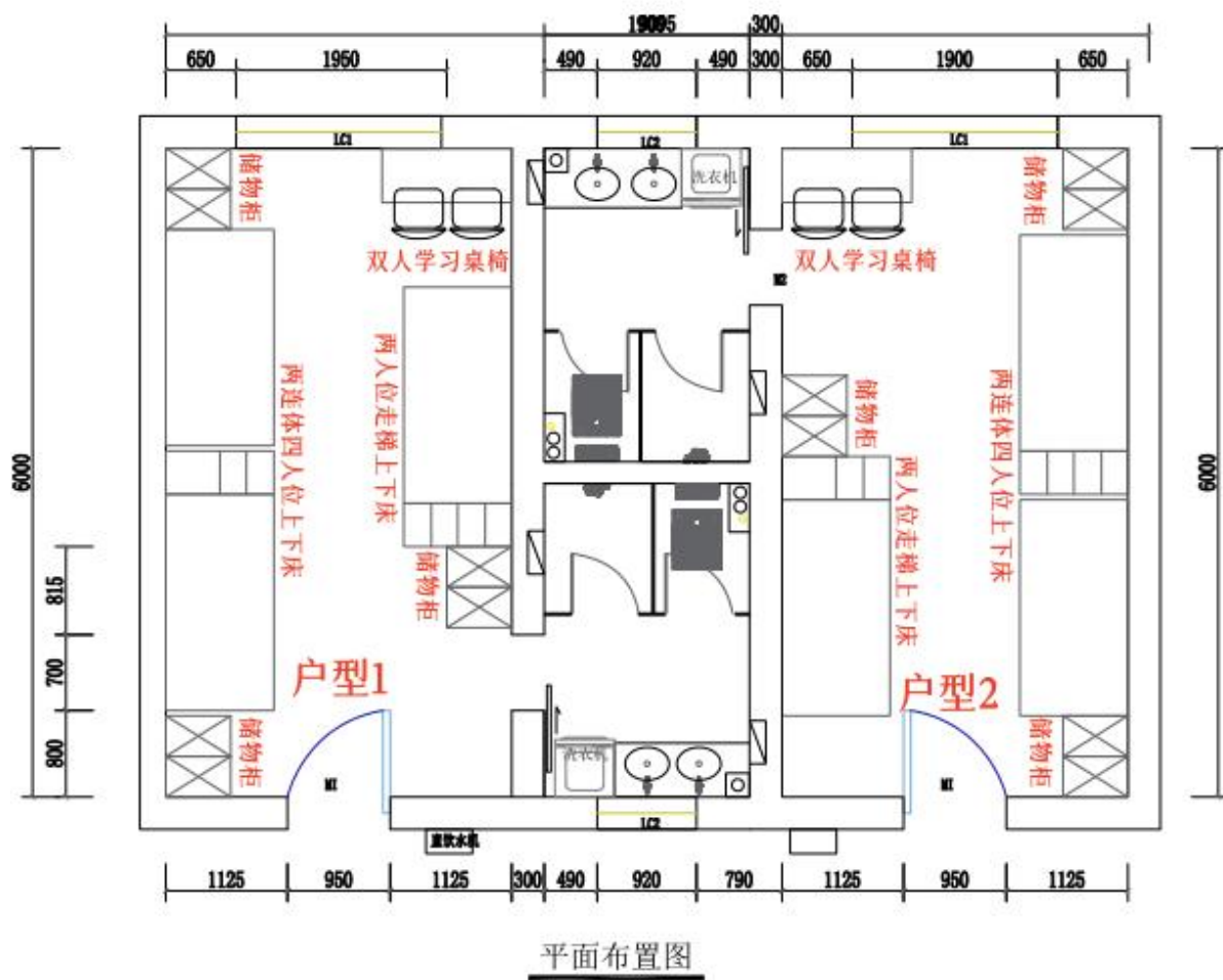
图 1：宿舍户型平面布置图
