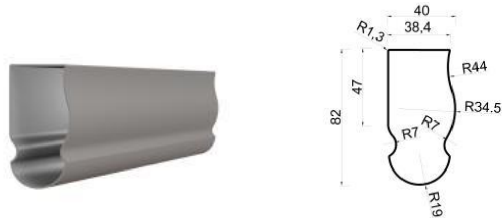
图 6：床横梁参考示意图
