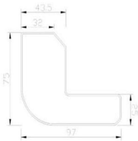
图 5：上下铺立柱参考示意图
