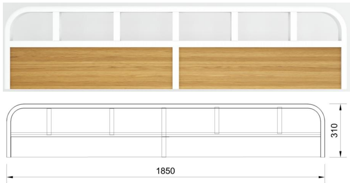
图 8：前护栏参考示意图
