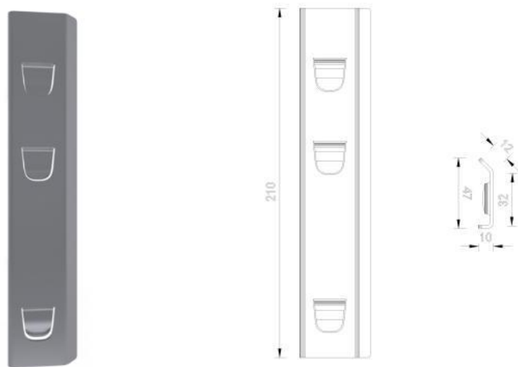
图 7：连接件参考示意图
